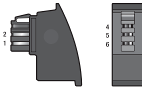
TAE/RJ45-Adapter: Pins des TAE-Steckers
