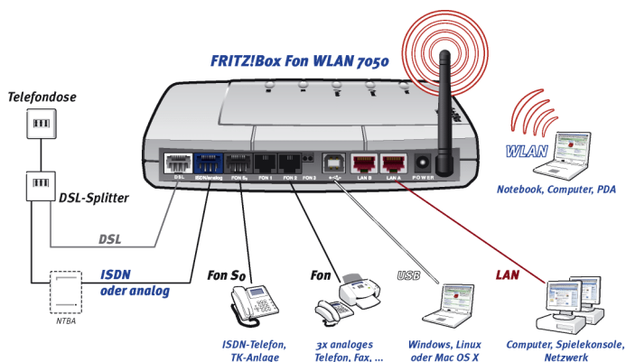
Anschlussmöglichkeiten der FRITZ!Box Fon WLAN
