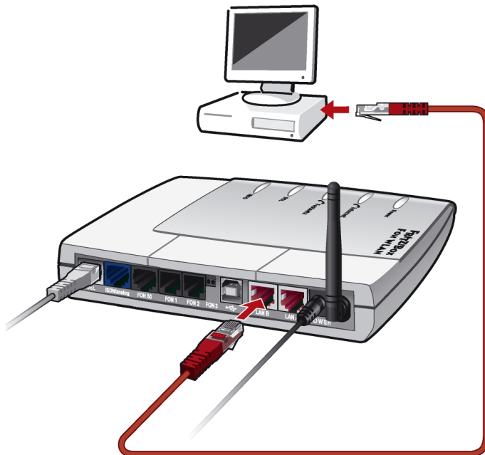
Anschluss eines Computers an einen Netzwerkanschluss der FRITZ!Box Fon WLAN
