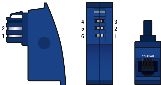
TAE/RJ45-Adapter seitlich, von vorn und Buchsenseite
