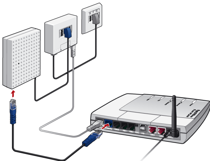
Anschluss der FRITZ!Box Fon WLAN am ISDN-NTBA
