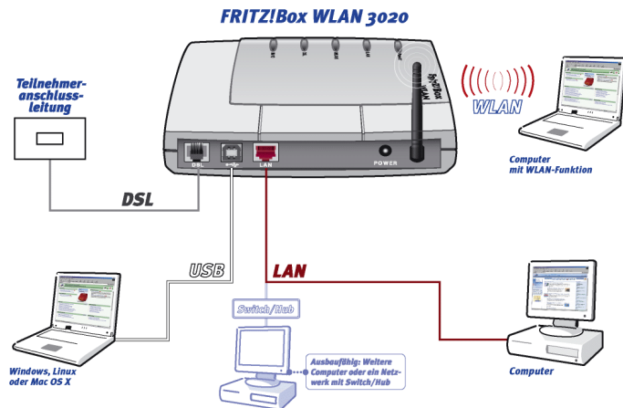
Anschlussmöglichkeiten der FRITZ!Box WLAN
