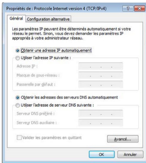
Propriétés du protocole Internet (TCP/IP)
